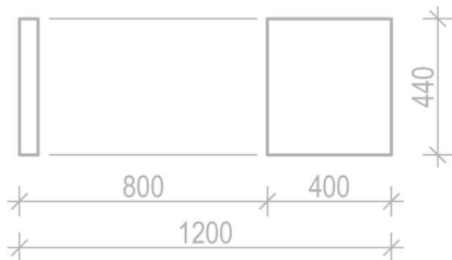
ansicht
