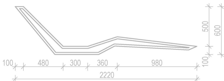
ansicht
